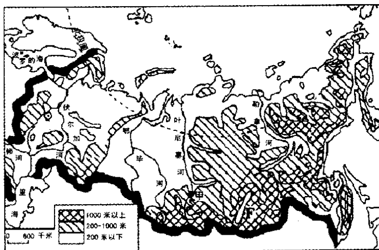
俄罗斯地形略图
