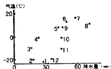
甲地各月多年平均气温和降水量
