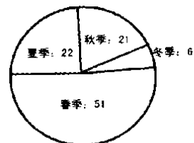
叶尼塞河各季径流占全年径流量 (%)
