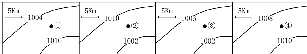
四地等压线分布示意图（单位：hpa）
