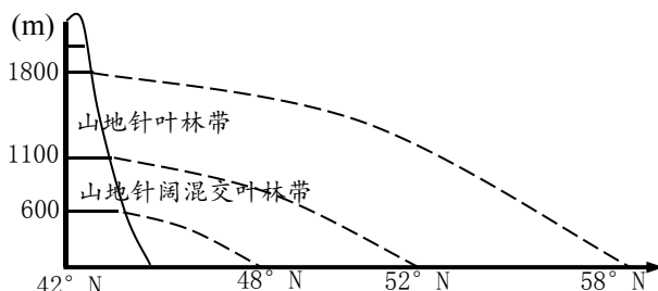
北纬 42° 某山地部分垂直自然带 与水平自然带对应关系示意图
